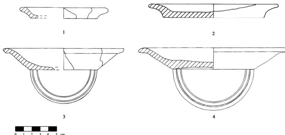
Fig. 15. Piattelli: 1. piattello 1 II 1; 2. piattello 1 II 2; 3. piattello 1 IV 1; 4. piattello 1 IV 2 (disegni M.T.A. Robino).
