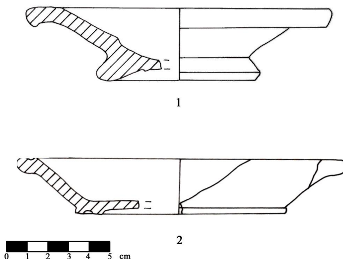
Fig. 16. Piattelli: 1. piattello 2 IV 2; 2 piattello 3 IV 2 (disegni M.T.A. Robino).
