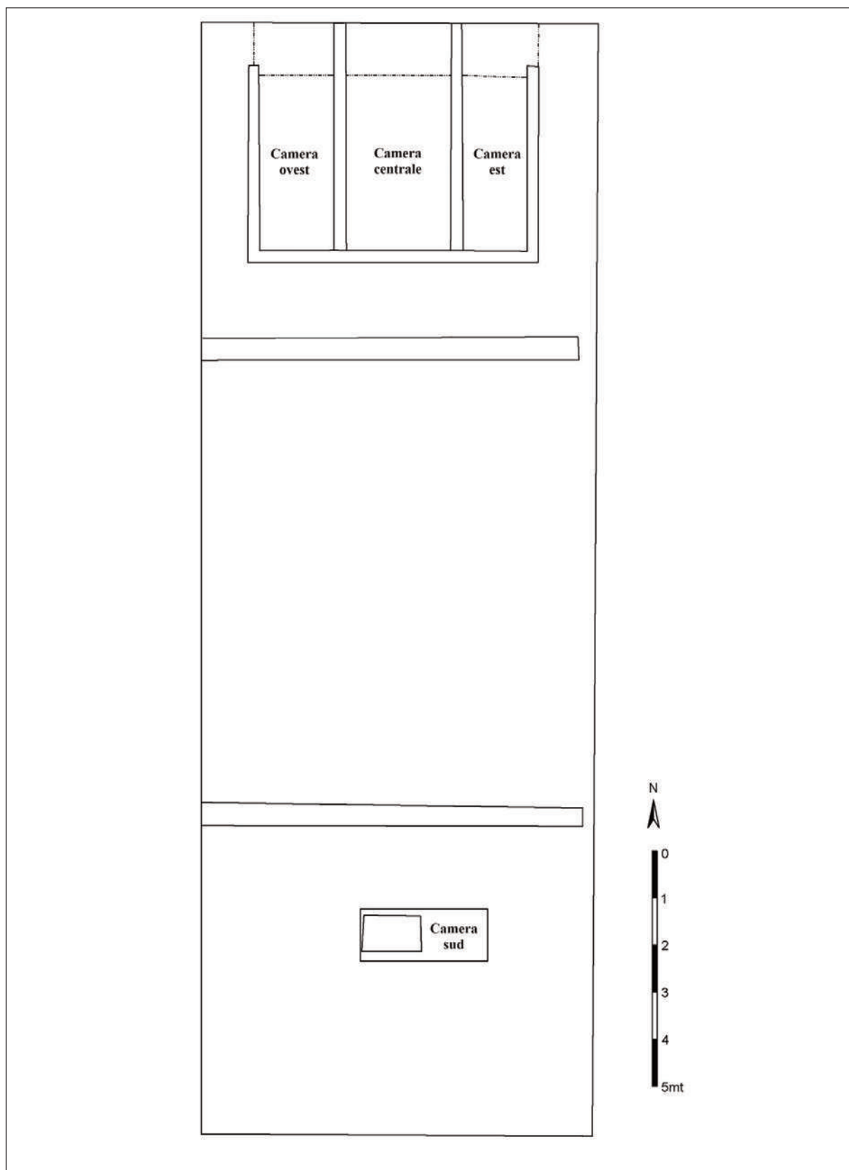
2. IL COMPLESSO DELL'EX CONVENTO DI SAN NICOLAO A LUCCA: PIANTA SCHEMATICA DELL'AMBIENTE NORD-ORIENTALE CON POSIZIONAMENTO DEI VANI IPOGEI (rilievo Francesco Coschino; Archivio SABAP-LU)
